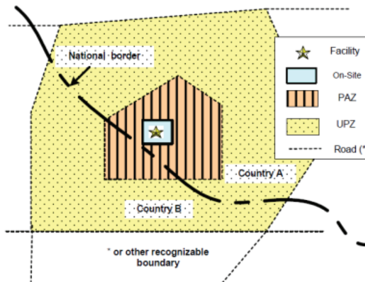
تصویر ۲-۵: حوزه‌های و زون‌های اضطراری (INES2017)
