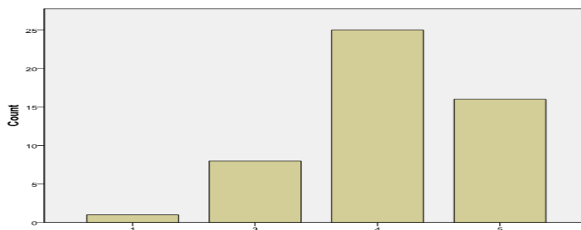
نمودار ۳: نمودار پراکندگی سؤال ۳۰
