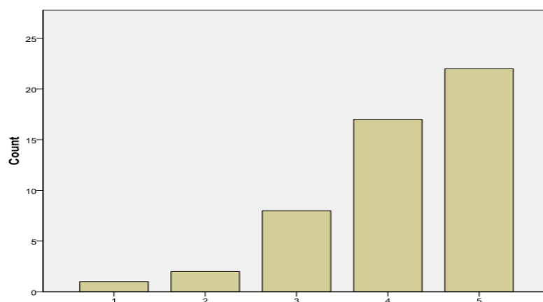
نمودار ۱: نمودار پراکندگی سؤال ۱۰
