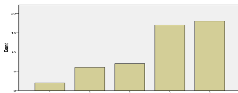
نمودار ۲: نمودار پراکندگی سؤال ۱۸
